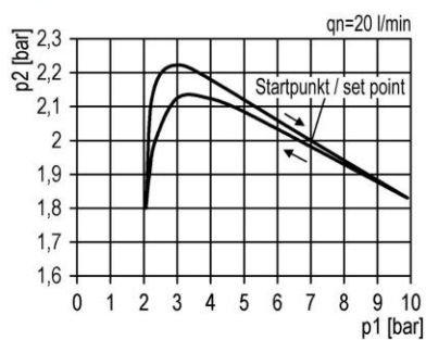
Hysterese
