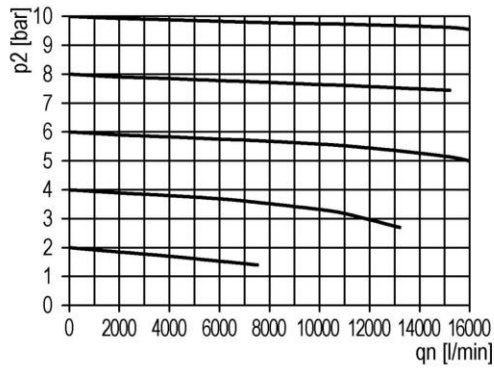
Durchflussdiagramm
