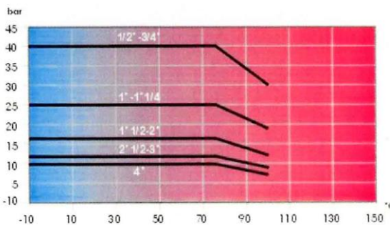
Druck-/Temperatur-Diagramm
